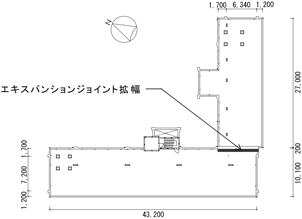
屋階平面図
