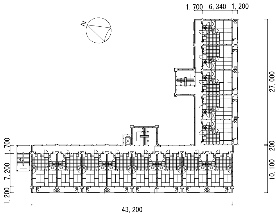
5 ～ 6 階 平 面 図
